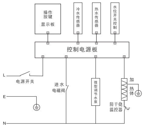
电器原理图
