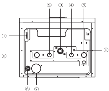
冷凝炉下接口尺寸
