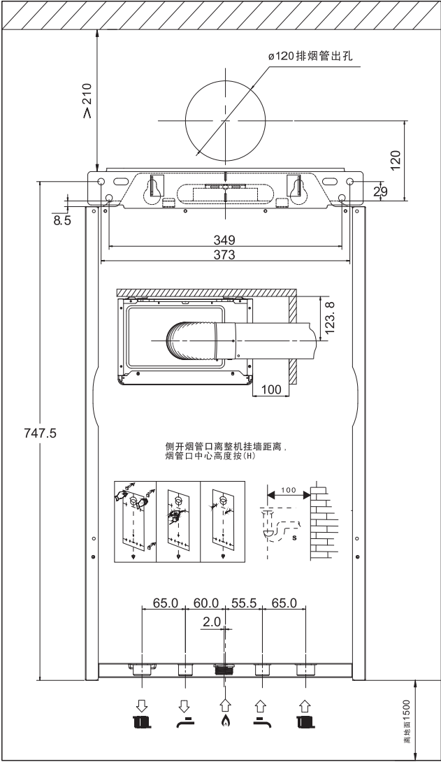
安装图样 (单位: mm)
