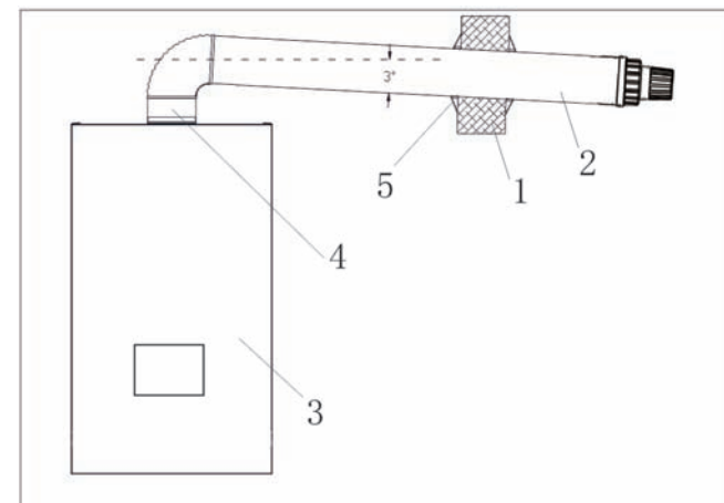
图5.5.2标配烟管的安装
