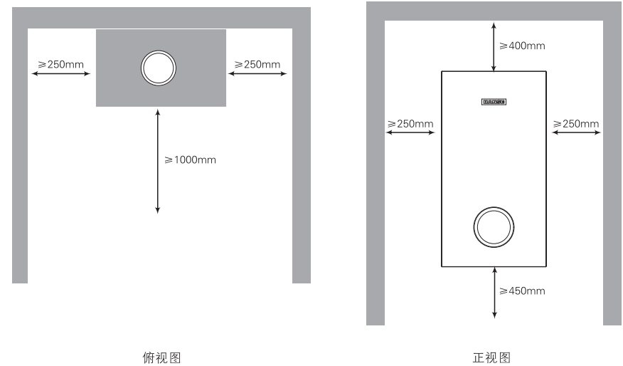
俯视图
