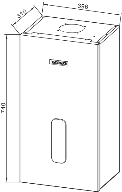
外型尺寸（mm）
