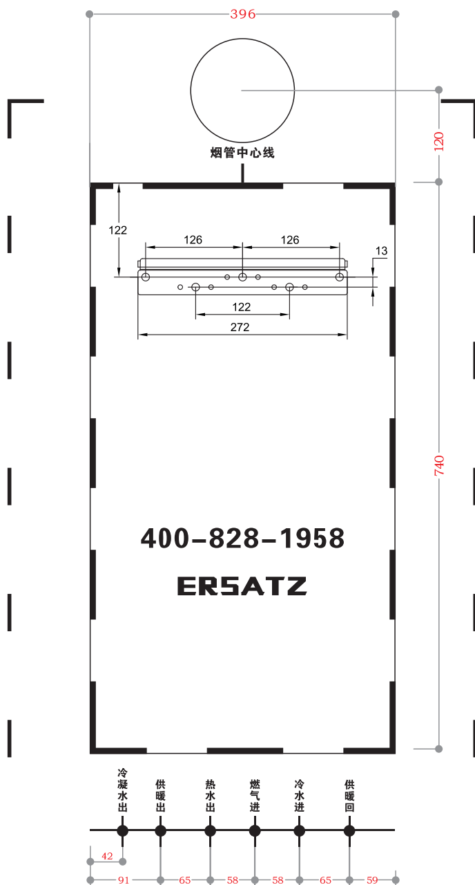
安装定位尺寸 (mm)
