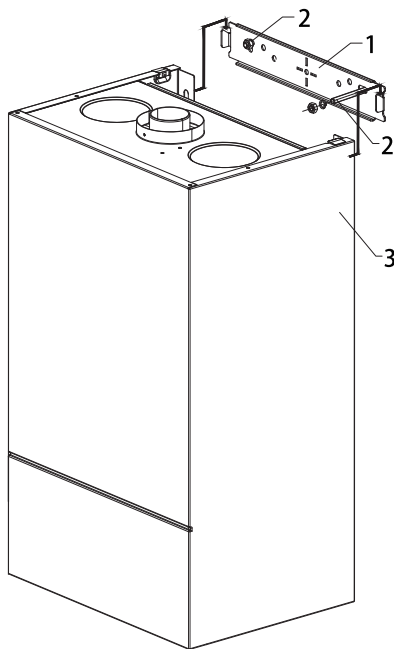
图4.6采暖炉的安装（具体请参照实机及附件）
