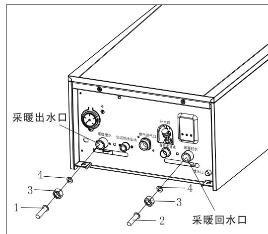
图5.4.1采暖系统出/回水管路的连接
