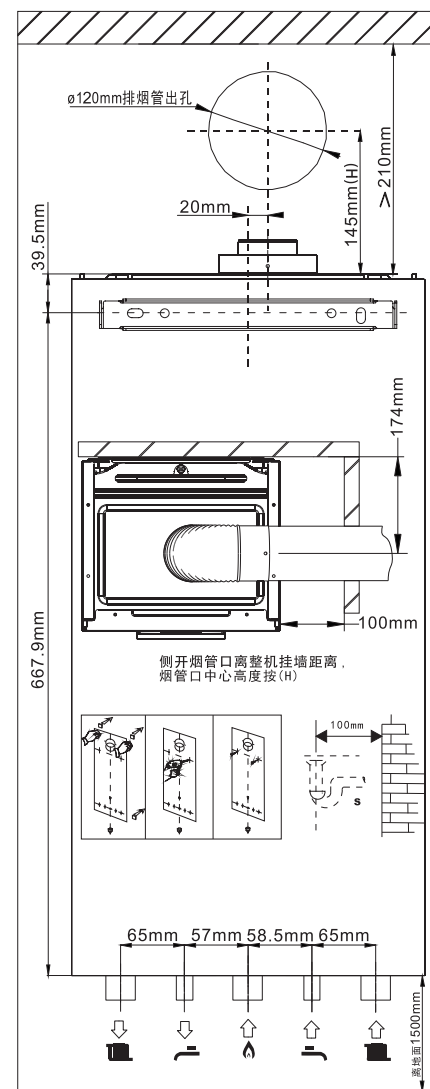
安装图样
