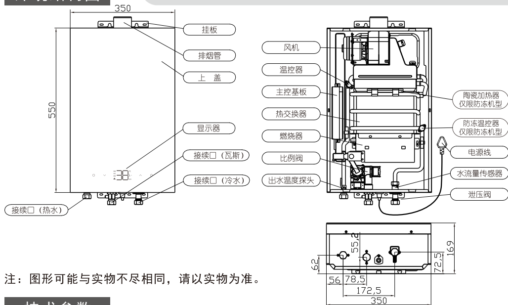
外观结构图
