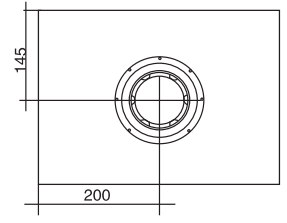
炉顶部进排烟口俯视图（φ 80/125）
