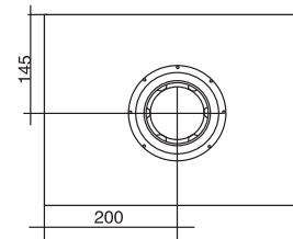
炉顶部进排烟口俯视图（ \varnothing 80/125 ）
