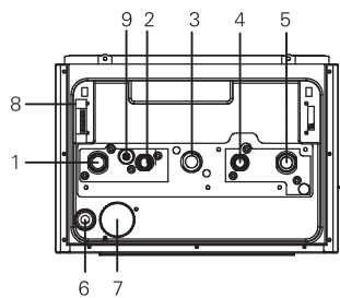
冷凝炉下接口尺寸
